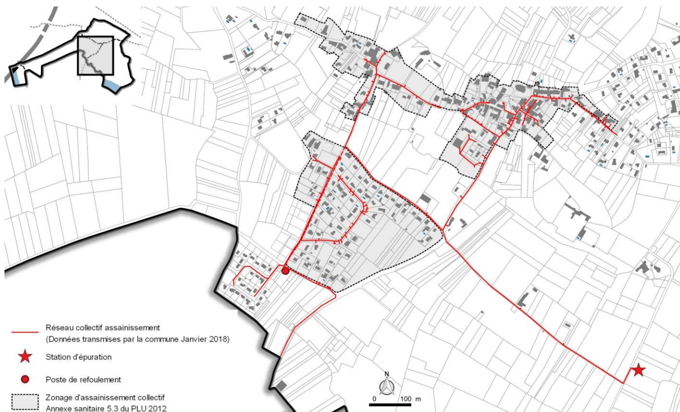
Schématisation du réseau d'assainissement sur la commune
